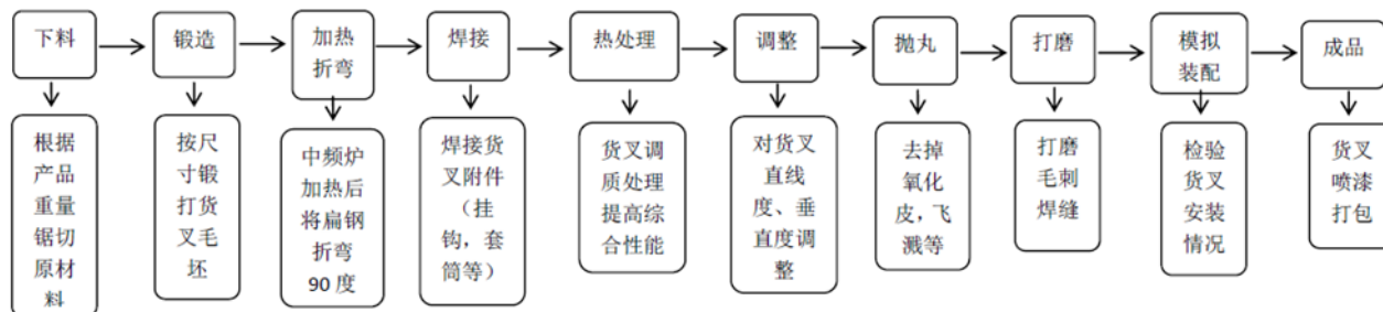
图 3-2 锻造货叉工艺流程图
