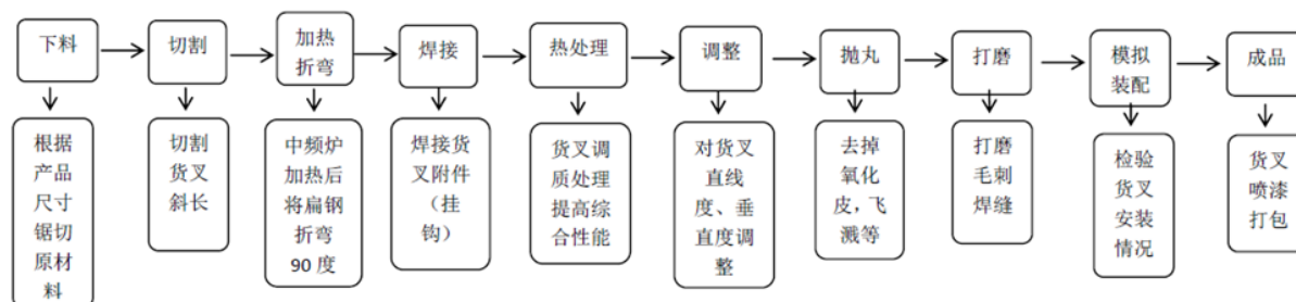
图 3-1 型材货叉工艺流程图
